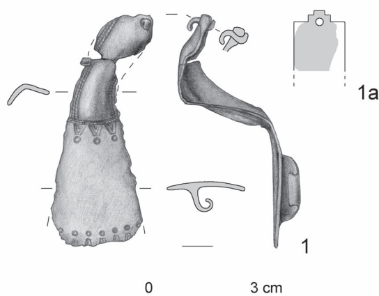
Rycina 1. Szwałk, st. 18. Zapinka brązowa: 1. Rysunek zapinki; 1a. Rekonstrukcja kształtu główki. Rys. A. Grzędzińska, P. Szymański
