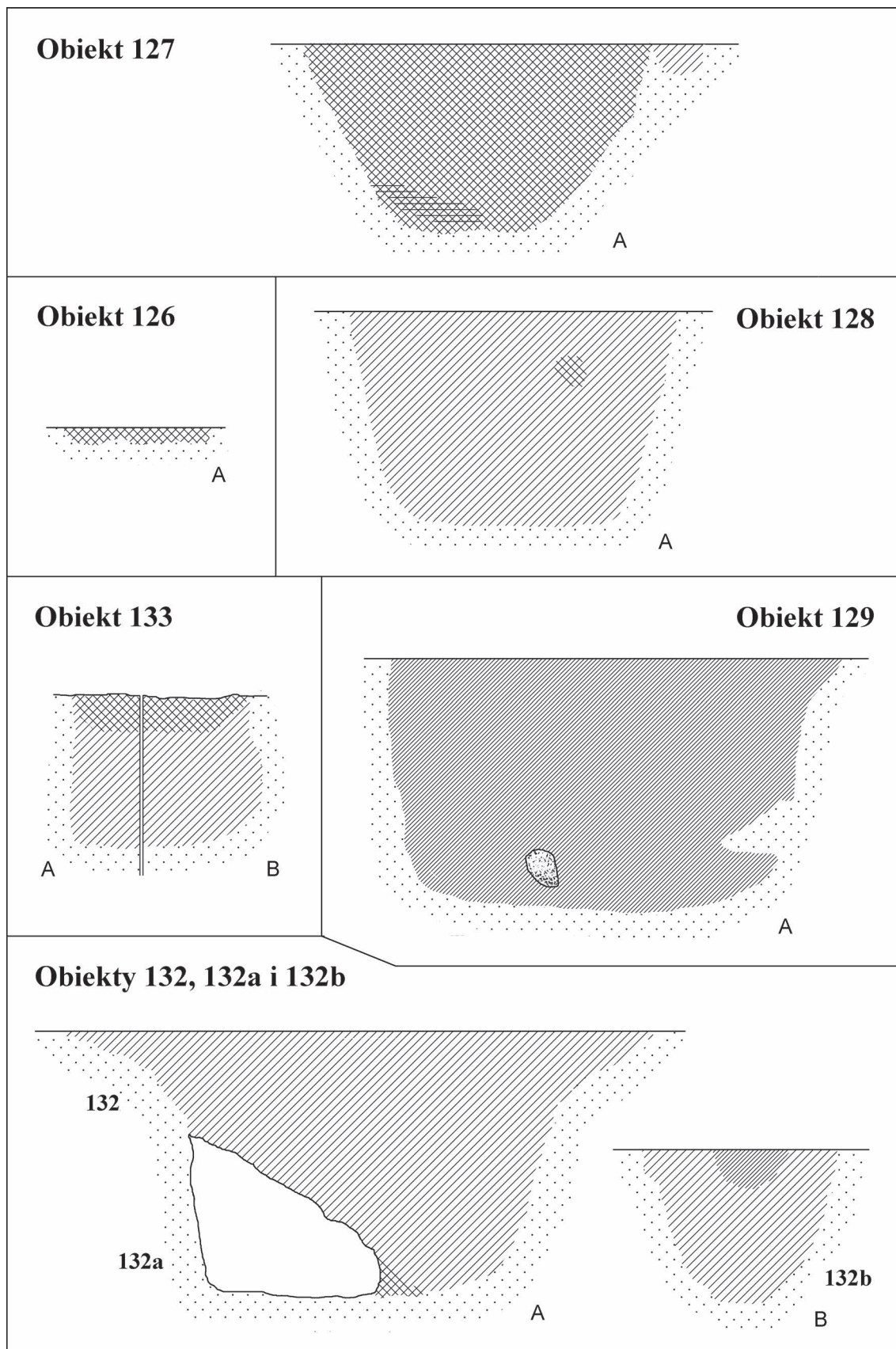
Tablica LI. Tworki Skrodzkie, st. I. Obiekty 126–129, 132, 132a, 132b, 133. Obiekt 133: A. profil E obiektu, B. profil S obiektu. Opr. A. Bucholc
